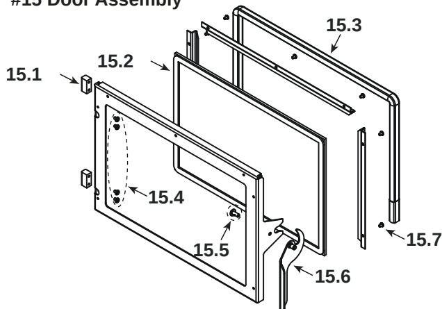
#15 Door Assembly
